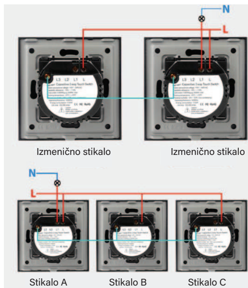
Trojno izmenično stikalo
