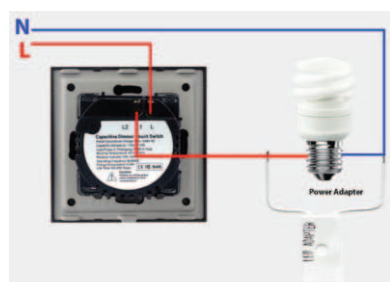
Trojno izmenično stikalo
