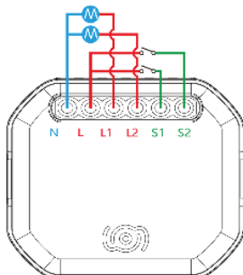
Wi-Fi modul za stikalo za rolete in zaves
