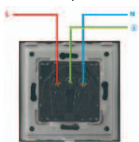
Vtičnica tipa F
