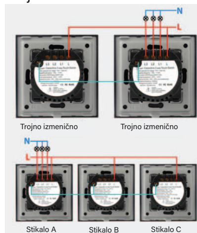
Trojno izmenično stikalo
