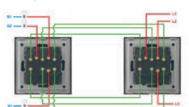
Trojno izmenično stikalo
