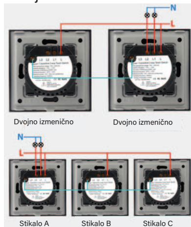
Dvojno izmenično stikalo
