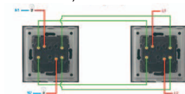
Enojni križno stikalo
