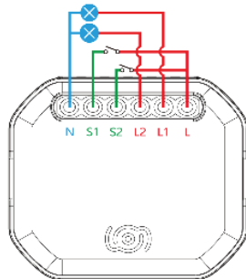
Wi-Fi modul za dvojni zatemnilnik
