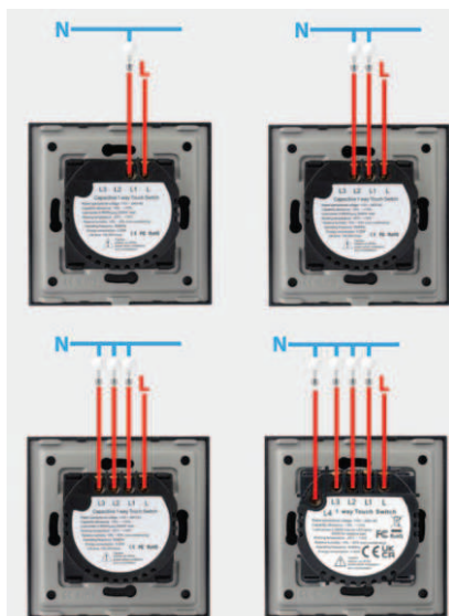
Stikalo na dotik
