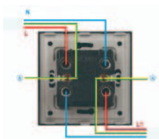
20A/45A Dvopolno stikalo
