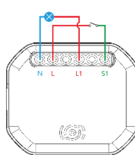
Wi-Fi modul za enopolni zatemnilnik
