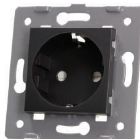
MODUL UTIČNICA CRNA BOJA KATALOŠKI BROJ WG-71 EU-62 DIMENZIJE: 45 * 45 mm Napon: 110 V-250 V / 50 Hz-60 Hz Struja: 10 A Radno okruženje: -30 ~ 70 ° C
