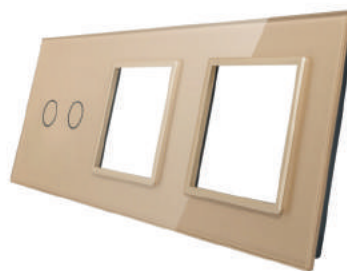
PANEL ZA PREKIDAČ 1 + DUPLI OKVIR ZLATNA METALIK BOJA KATALOŠKI BROJ 702GG-63 DIMENZIJE: 222mm*80mm*4mm UGRADNJA: EU stand. okrugla trostruka kutija Ø 60 mm
