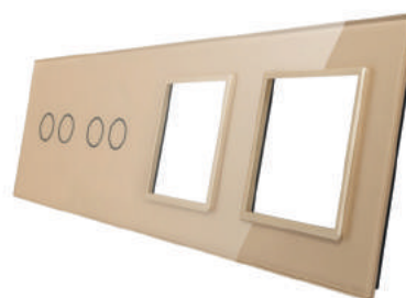
PANEL ZA PREKIDAČ 2 + 2 OKVIRA ZLATNA METALIK BOJA KATALOŠKI BROJ 7022GG-63 DIMENZIJE: 293mm*80mm*4mm UGRADNJA: EU stand. okrugla četvorostruka kutija Ø 60 mm
