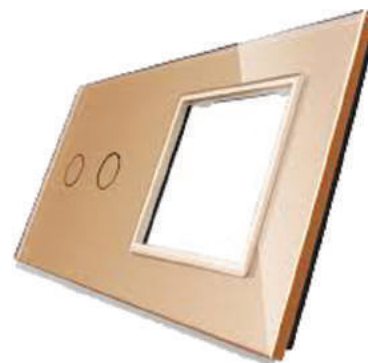
PANEL ZA PREKIDAČ 2+ OKVIR ZLATNA METALIK BOJA KATALOŠKI BROJ 702G-63 DIMENZIJE: 151 mm*80 mm*4 mm UGRADNJA: EU stand. okrugla dvostruka kutija Ø 60 mm
