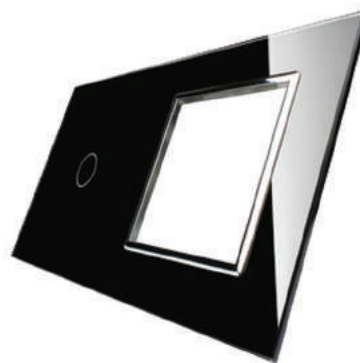
PANEL ZA PREKIDAČ 1+ OKVIR CRNA BOJA KATALOŠKI BROJ 701G-62 DIMENZIJE: 151mm*80mm*40mm BIJEŠKA: EU stand. okrugla dvostruka kutija Ø 60 mm
