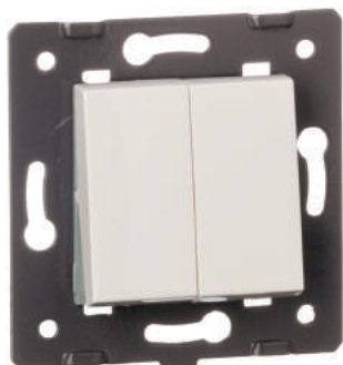
MODUL IZMJENIČNI DVOSTRUKI PREKIDAČ KATALOŠKI BROJ 1FKS-61 DIMENZIJE: 2*modul 22,5mm Radni napon: izmjenična struja 110 V-250 V / 50 Hz-60 Hz Jakost električne struje: 10A
