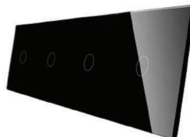
PANEL ZA PREKIDAČ 1+1+1+1 CRNA BOJA KATALOŠKI BROJ 701111-62 DIMENZIJE: 293mm*80mm*4mm UGRADNJA: EU stand. okrugla četvorostruka kutija Ø 60 mm
