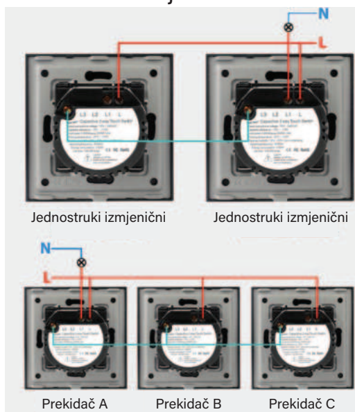
Trostruki izmjenični
