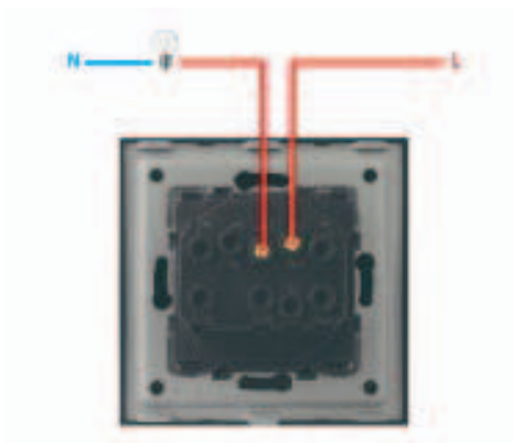
Jednopolni prekidač
