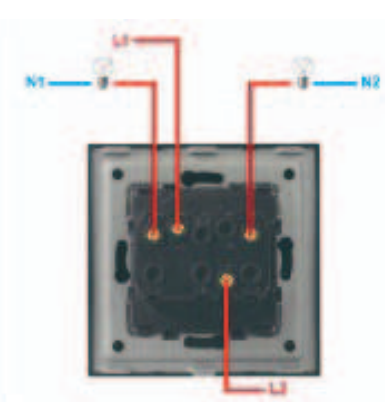
Serijski prekidač
