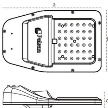
Tehnički prikaz dimenzija:
