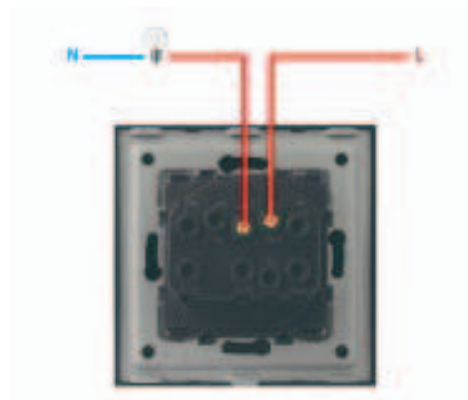
Jednopolni prekidač
