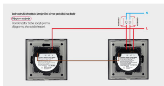
Jednostruki/dvostruki dimer
