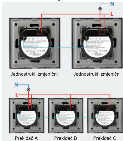
Trostruki izmjenični
