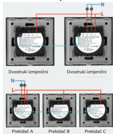
Dvostruki izmjenični
