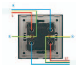
20A/45A Dvopolni prekidač
