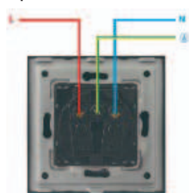
Tip F utičnica
