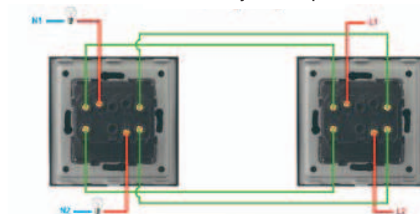
Jednostruki križni prekidač
