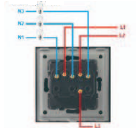
Trostruki prekidač
