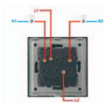
Serijski prekidač
