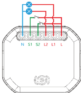
Wi-Fi modul za dvostruki dimer
